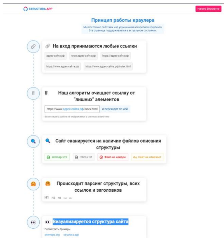
Рисунок 28 – принцип работы краулера
