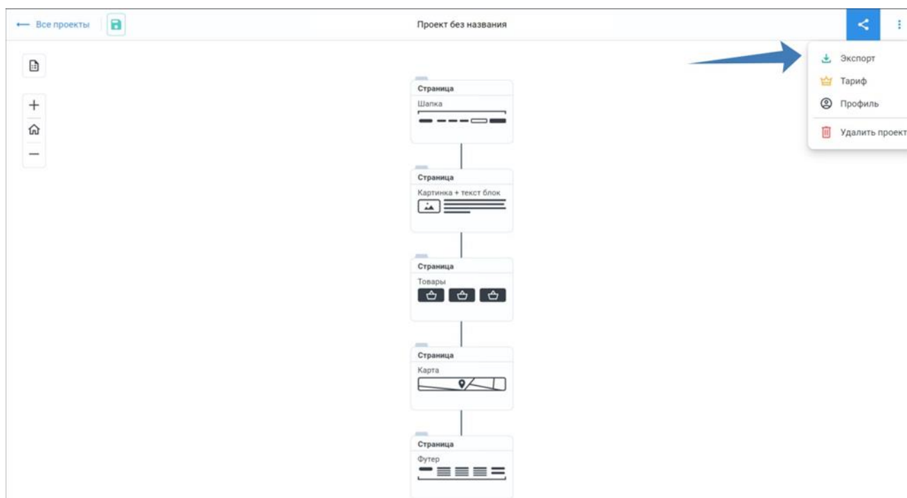
Рисунок 25 – экспорт проекта
