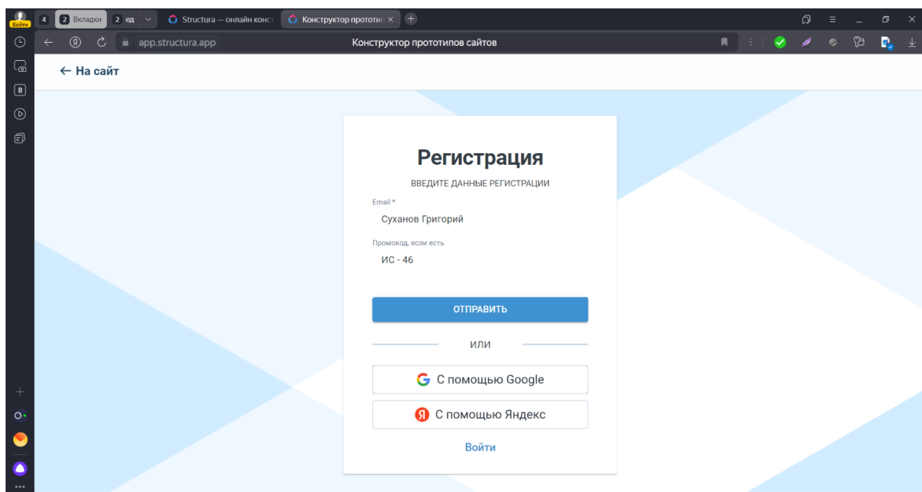
Рисунок 3 – форма регистрации
